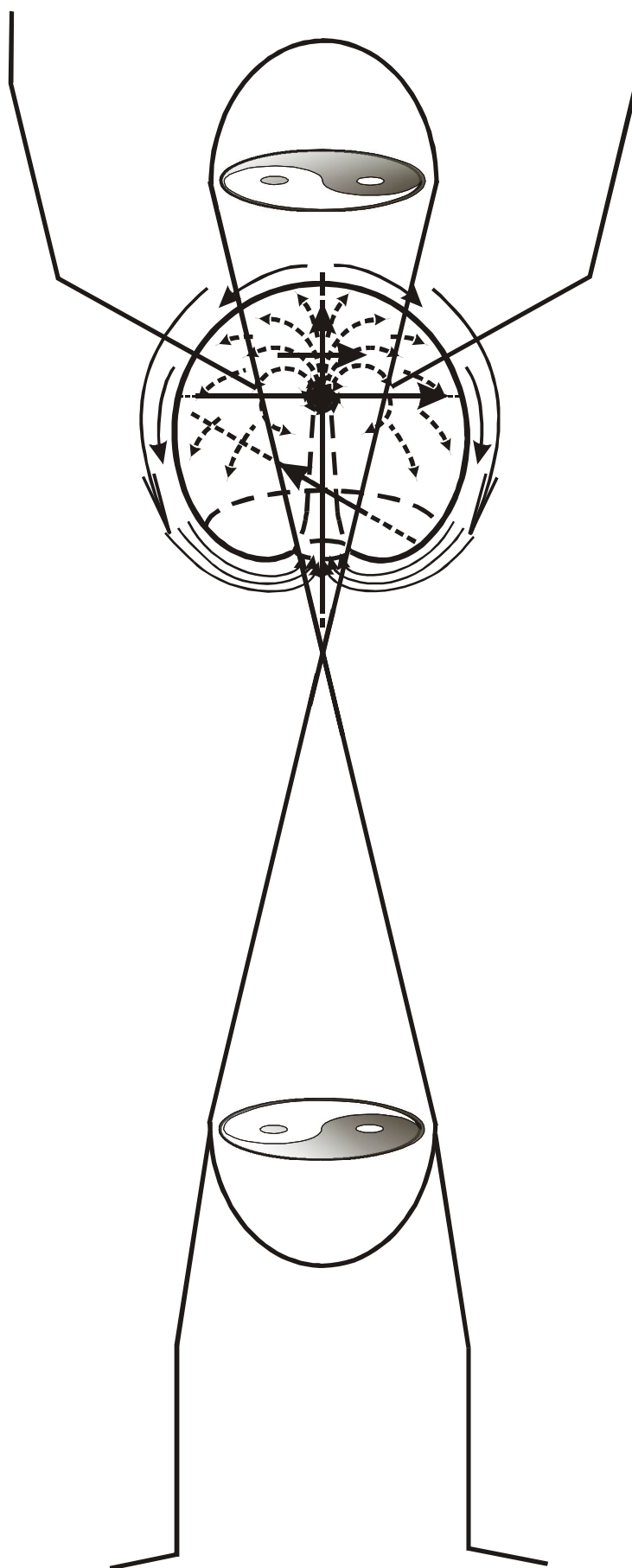
Рисунок 23 . Человек - существо космическое. В структуре и функции сердца человека повторяется основная схема строения Вселенной.
