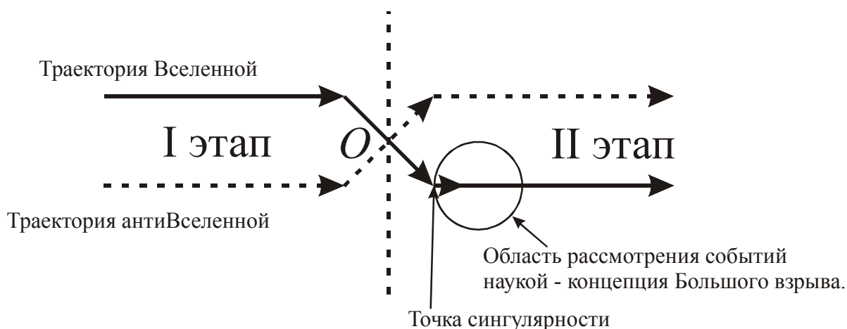
Рисунок 41. Взаиморасположение параллельных Вселенных
