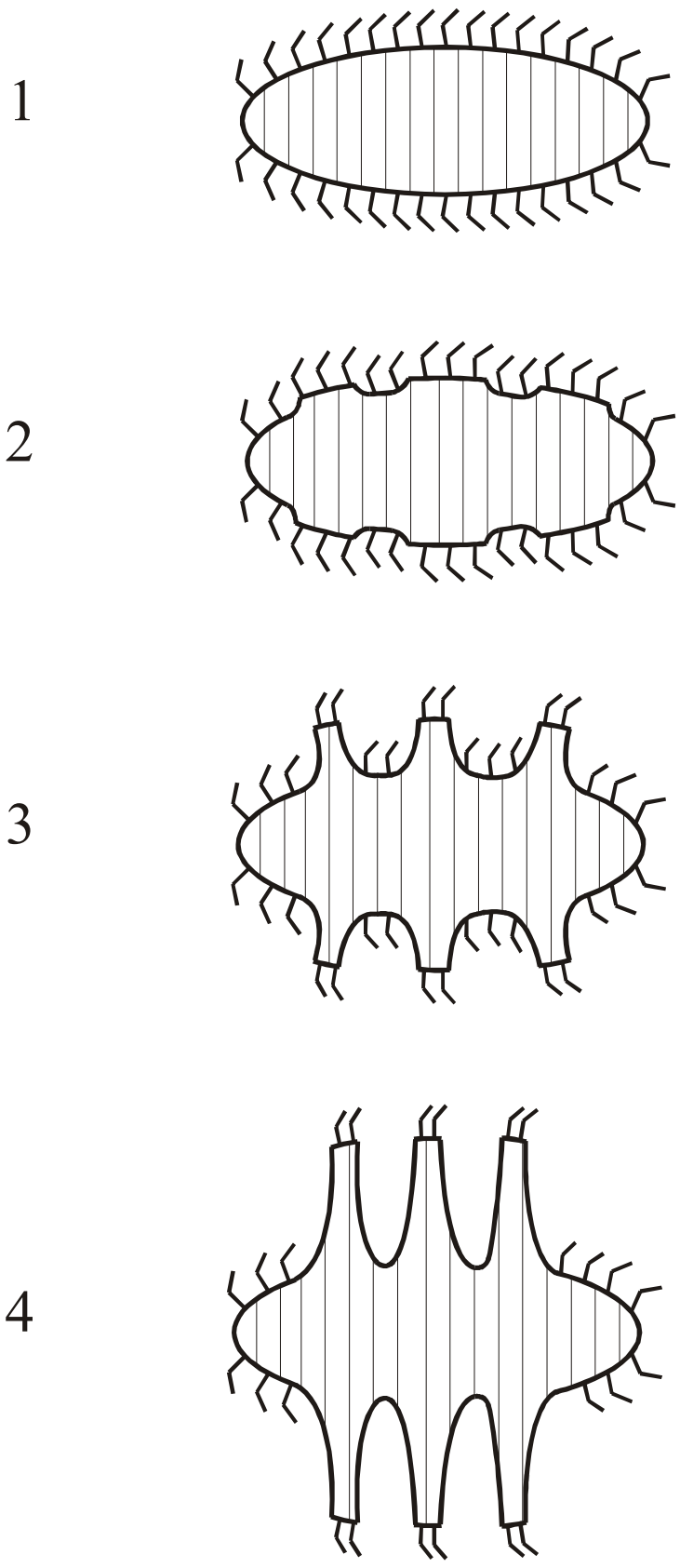
Рисунок 13. Процесс образования конечностей у насекомых.
