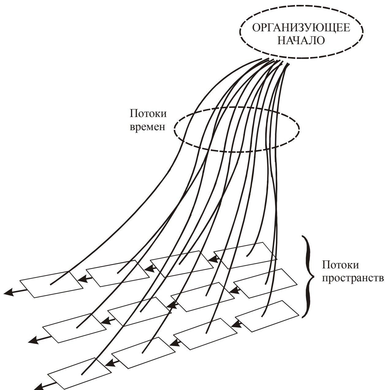
Рисунок 52. Потоки времен формируют потоки пространств.
