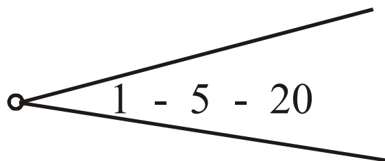
Рисунок 37. Вселенная находится в фокусе мироздания
