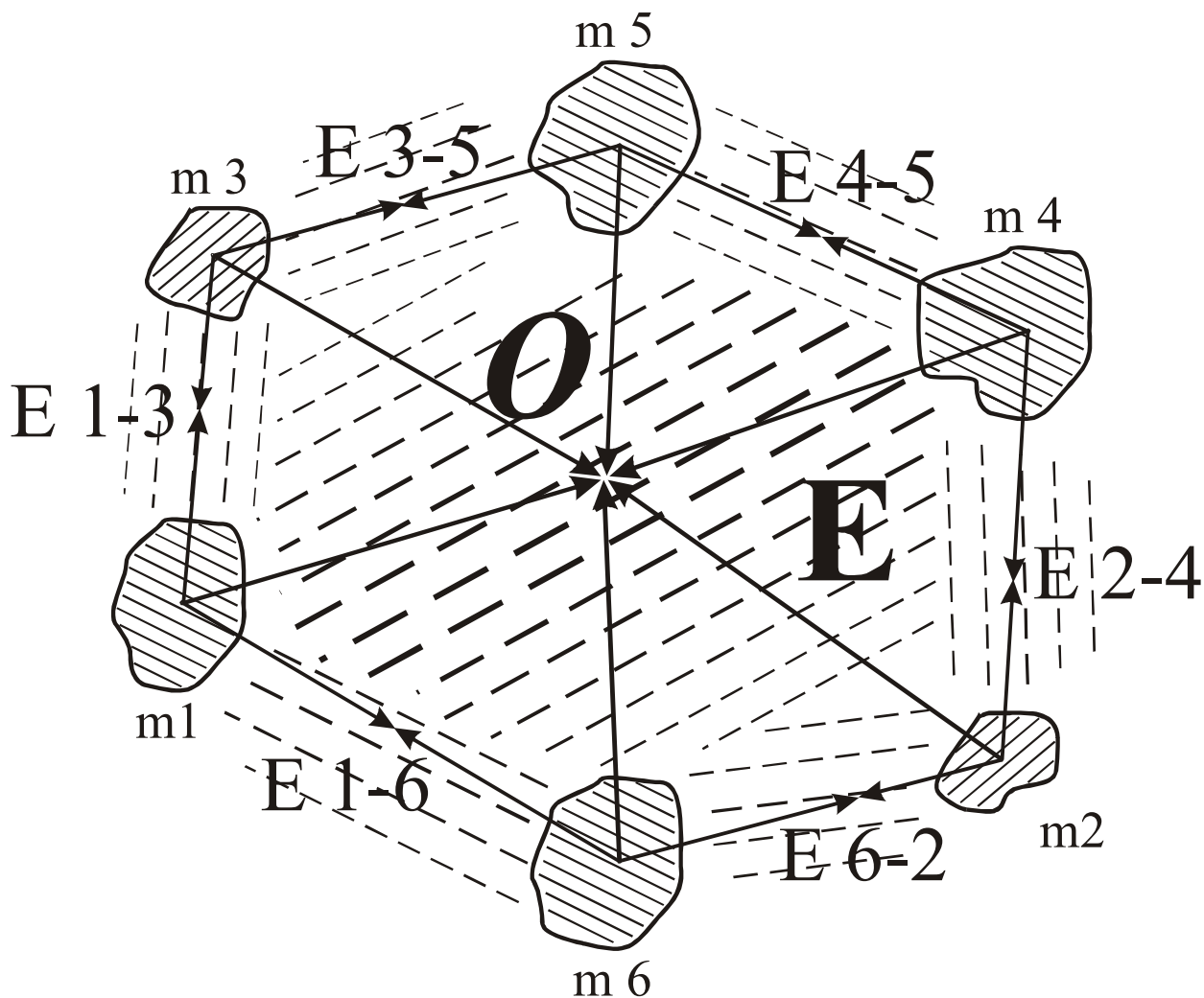
Рисунок 62. В итоге мироздание сформировалось как система тел, связанная результирующим полем E сложной формы и неравномерной плотности.
