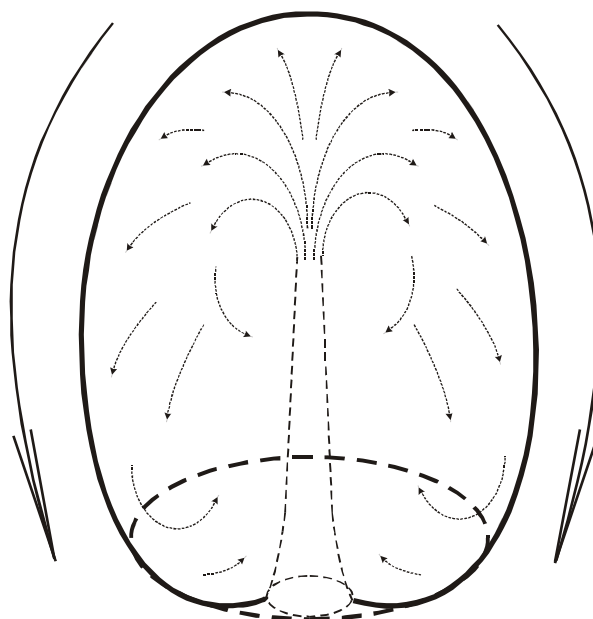
Рисунок 49. Циркуляция потоков энергии и вещества в космическом "яйце".
