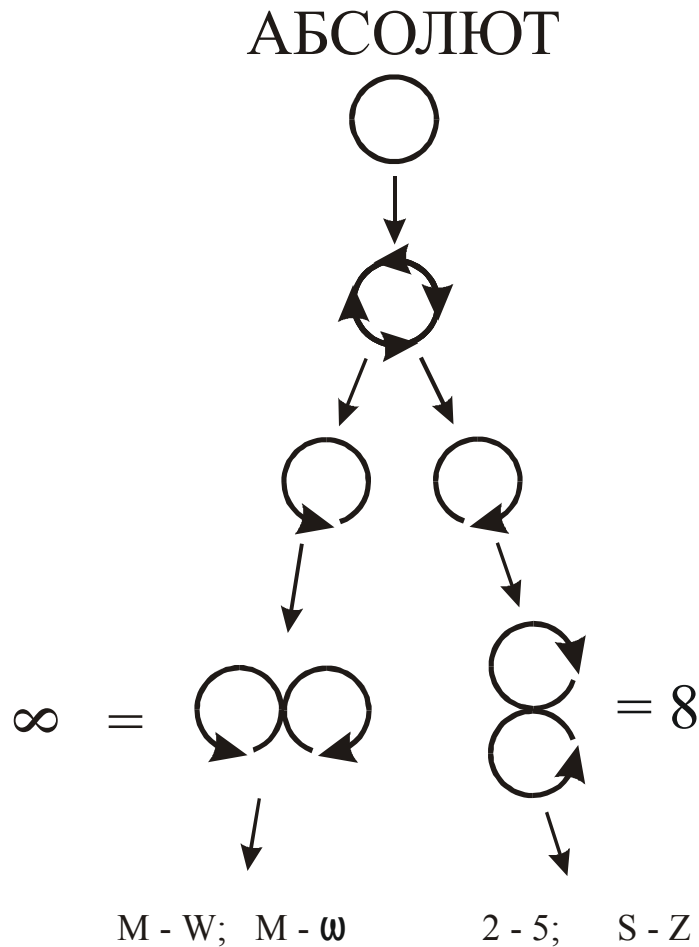
Рисунок 39. Принцип порождения парности: все структуры мироздания Абсолют созидает парами.
