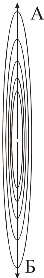
Рис. 14. Схема неограниченного роста тела человека
