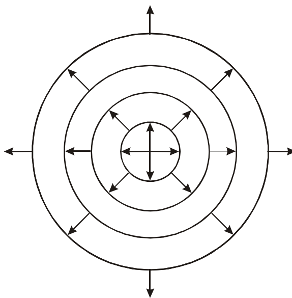
Рисунок 25. Структура слоев мироздания.
