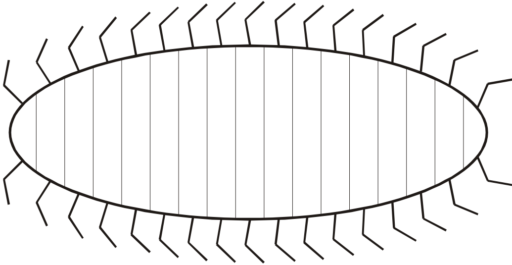
Рисунок 7. Сегментарное строение многоклеточных организмов. Модификация жгутиков.
