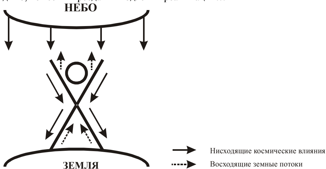
Рисунок 33. В древнем Китае человек изображался стоящим на Земле с воздетыми к Небу руками: так изображалась связующая роль человека - проводника воли Неба на Земле.
