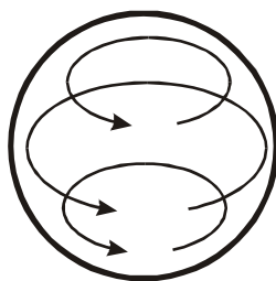
Рисунок 50. Элементарный модуль пространства.
