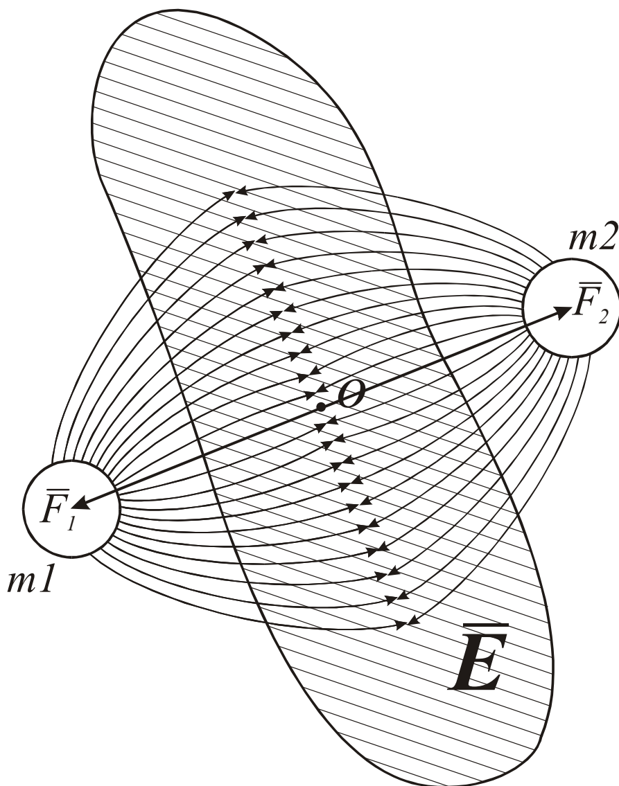
Рисунок 60. Притяжение масс m_1 и m_2 друг к другу - всего лишь иллюзия. В действительности каждая из них испытывает притяжение со стороны родительского поля E . Поле E - сложного, составного характера.
