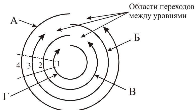
Рисунок 55. Механизм участия времени - системы двойной индексации объектов - в организации событий мироздания.
