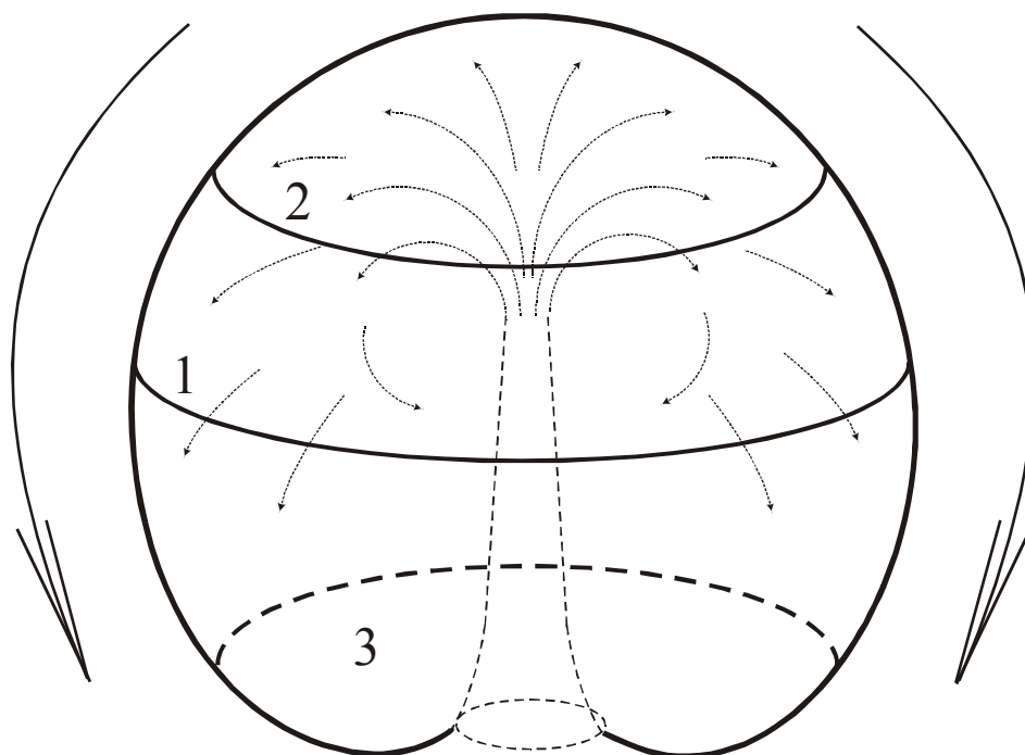
Рис. 20. Структура сложной системы “Земля”. 1 - экватор, 2 - 30-я параллель, 3 - область утилизации.
