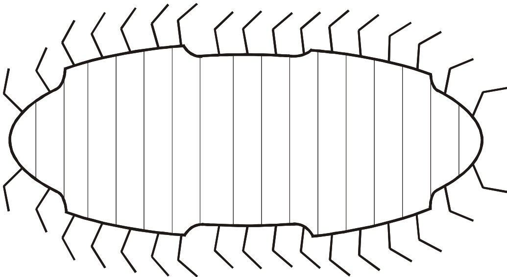
Рисунок 8. Начальный этап организации органов движения. Выделение симметричных фрагментов сегментов, несущих жгутики.
