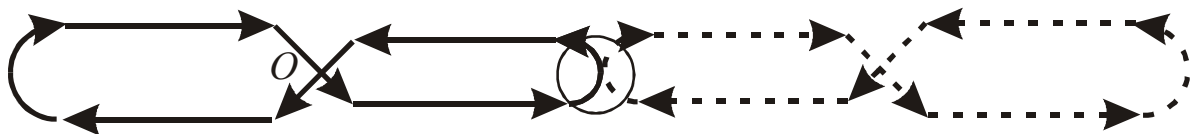
Рисунок 43. Циркуляция Вселенных вокруг общего центра. Вселенные выглядят как звенья цепи, или восьмерки.
