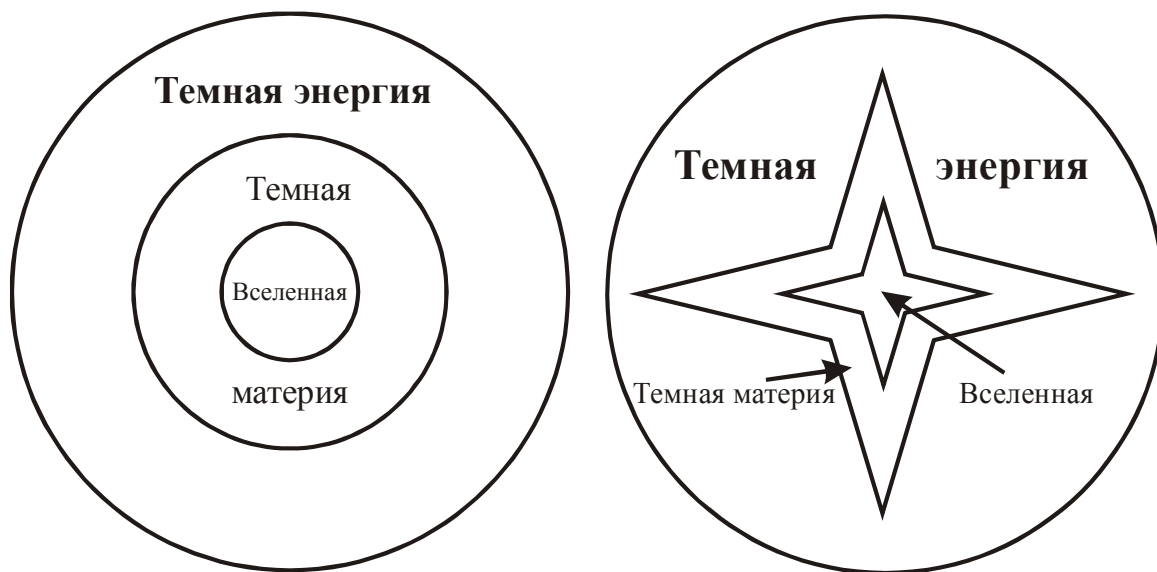
Рисунок 29. Пропорции вложенных миров.
