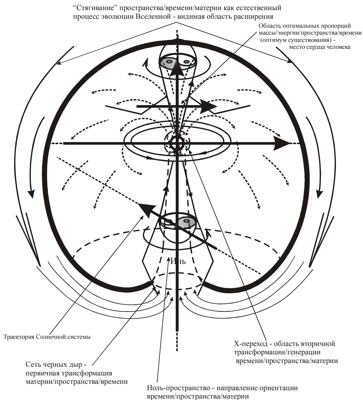
Рисунок 22. Человек - существо космическое - в его структуре и функции полностью повторяется основная схема строения мироздания.
