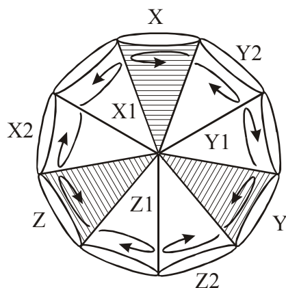
Рисунок 54. Сфера состоит из 9 конусов связанных в тройки пространств
