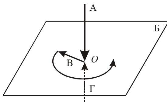
Рисунок 15. Механизм акцепции информации/энергии плоскостью.
