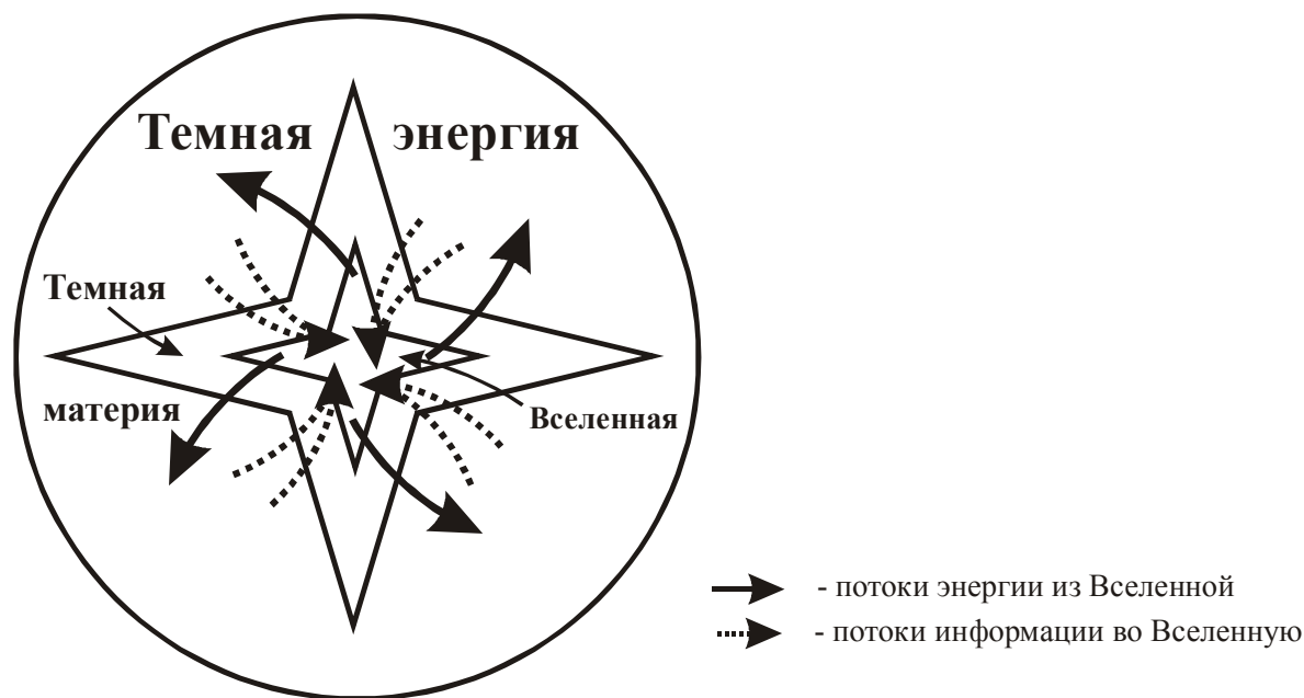
Рисунок 31. Информационные и энергетические связи Вселенной и мироздания.
