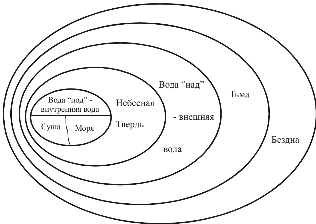
Рисунок 36. Пропорции составляющих компонент мироздания в терминах древних людей.
