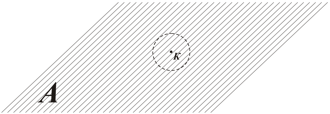
Рисунок 57. В поле континууме А будет сформирована частица в окрестностях точки К.
