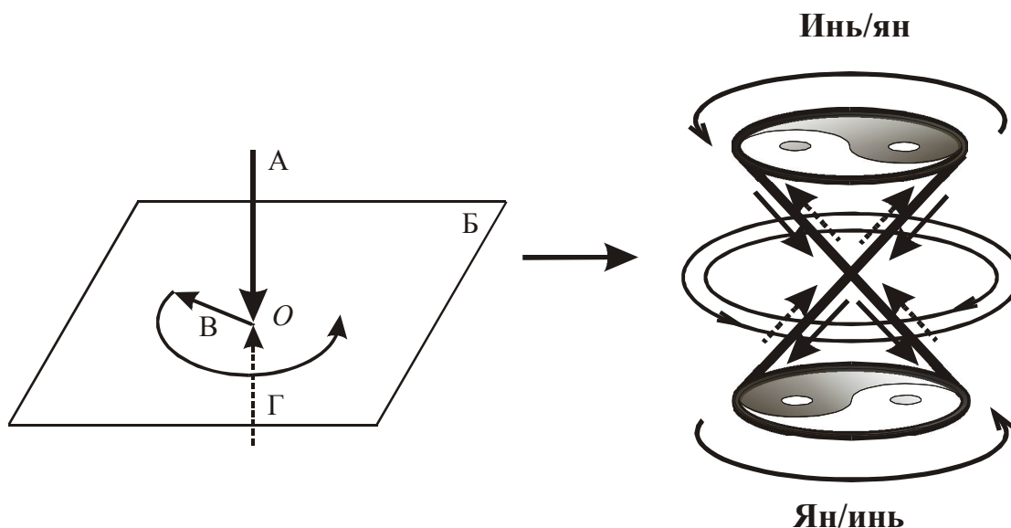
Рисунок 16. Концепция инь/ян и механизм излучения/акцепции.
