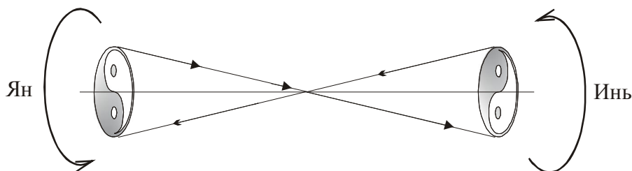
Рисунок 18. Истинный смысл монады Инь/Ян .
