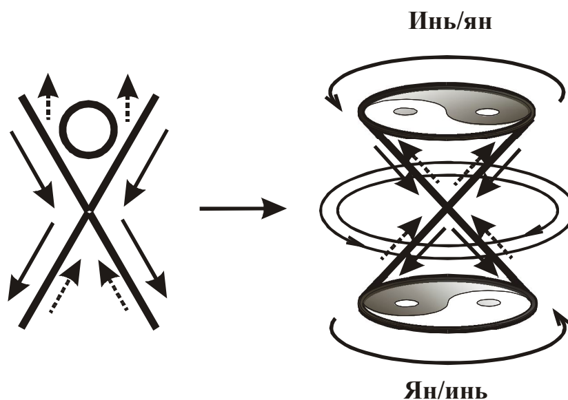
Рисунок 34. Человек реализован по схеме инь/ян. Сплошные стрелки - янская энергия, пунктир - иньская.
