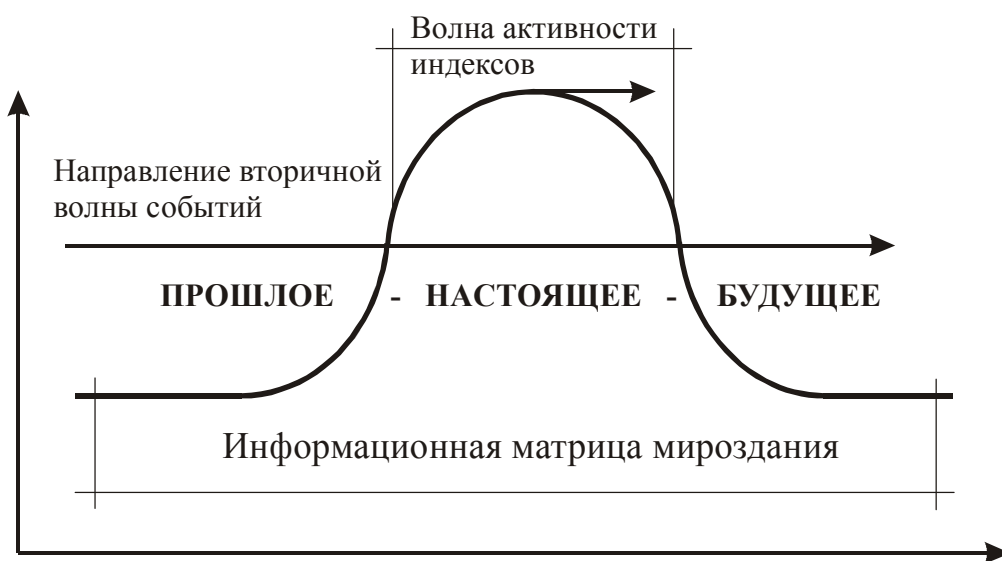
Рисунок 56. Организация потока событий в мироздании.
