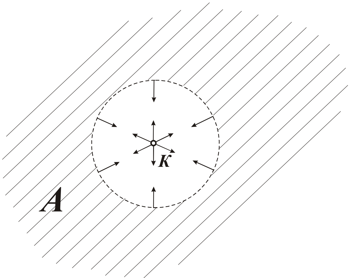
Рисунок 59. Содержимое фрагмента полевого континуума “стянуто” и преобразовано в частицу К. Континуум упруго восстанавливает свою целостность (стрелки направлены внутрь сферы).
