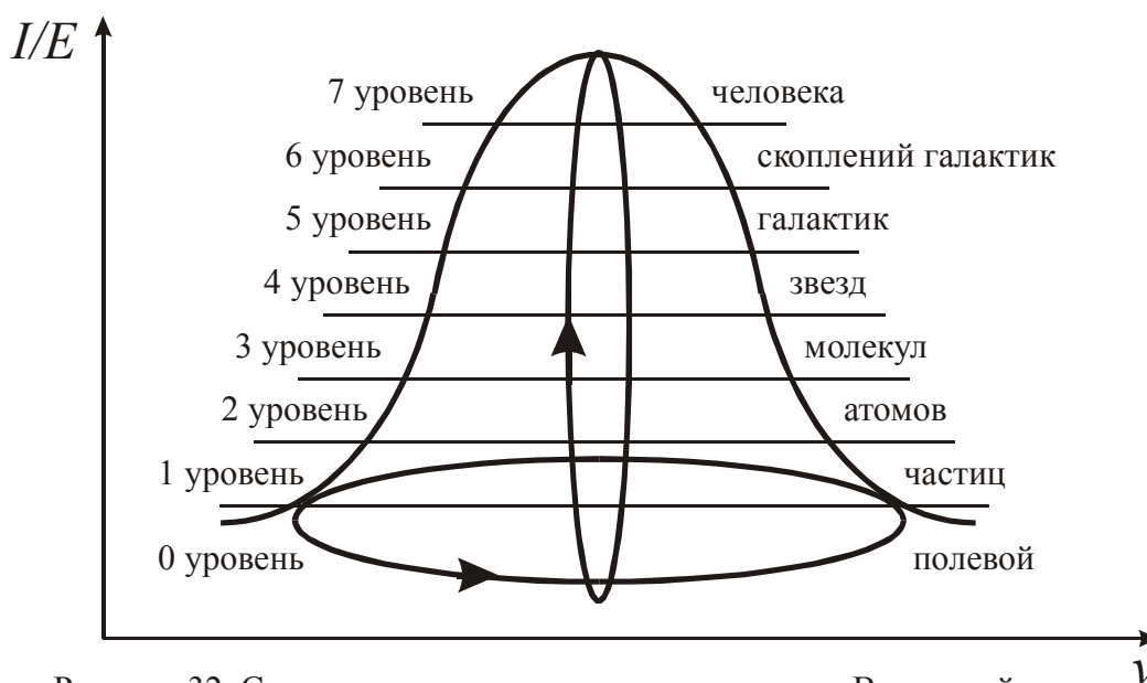
Рисунок 32. Симметрия жизненного цикла вещества Вселенной. I/E - информационно-энергетическое содержание уровня, v - объем уровня.
