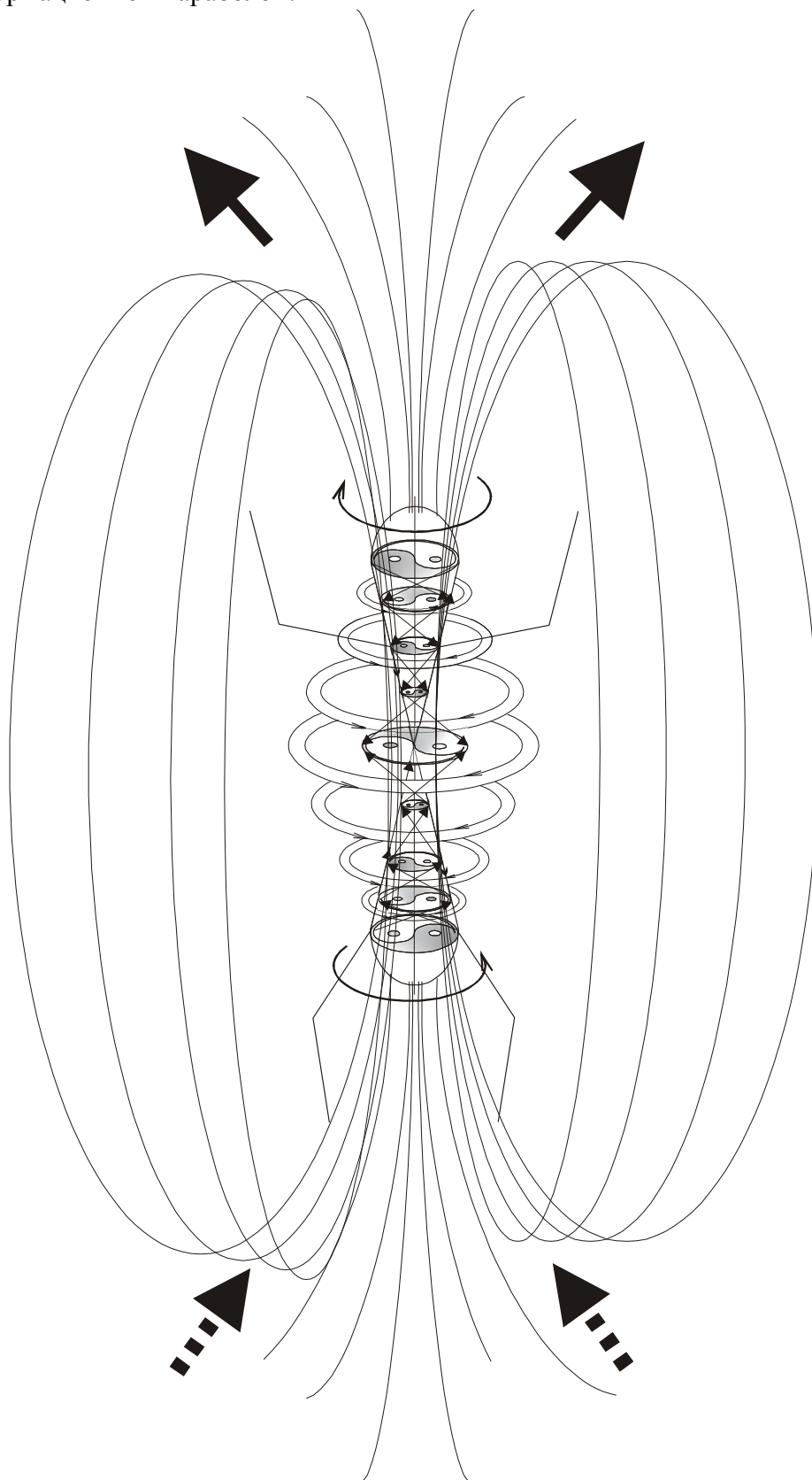
Рисунок 3. Человек - ходячий соленоид. Информационно-силовые линии поля человека сканируют бесконечность.
