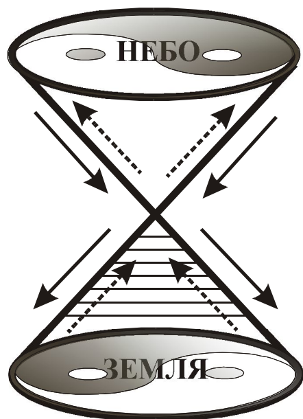
Рисунок 46. Небо, небесный порядок, увлекает и организует порядок земной. Показаны исходящие от Земли потоки обратной связи. Заштрихованная область - место человека..
