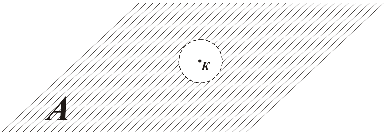
Рисунок 58. В точку К “стянуто” и преобразовано в частицу К содержимое полевого континуума, ограниченного окрестностями данной точки (показано пунктиром).
