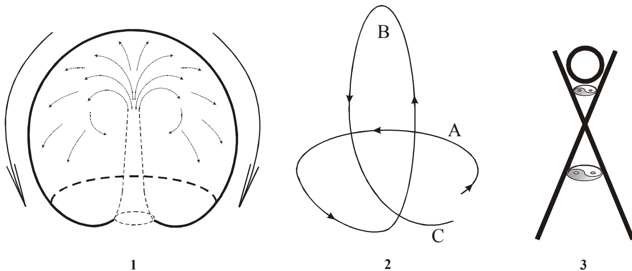
Рисунок 26. Общий принцип организации сложных систем. 1- схема циркуляции вещества, энергии и информации на планете Земля, во Вселенной и в мироздании; 2 - схема суточной циркуляции энергии в организме человека; 3 - в принципиальной схеме человека реализованы все принципы и схемы, свойственные сложным системам: и организм человека, и хромосомы построены по принципу пересечения потоков.
