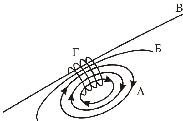
Рисунок 4. Схема типов человеческих судеб, пояснения в тексте.
