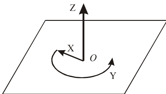
Рисунок 48. Развитие событий в плоскости (векторы X, Y) на первом этапе, и переход развития на следующий уровень - над горизонтом плоскости, вектор Z.
