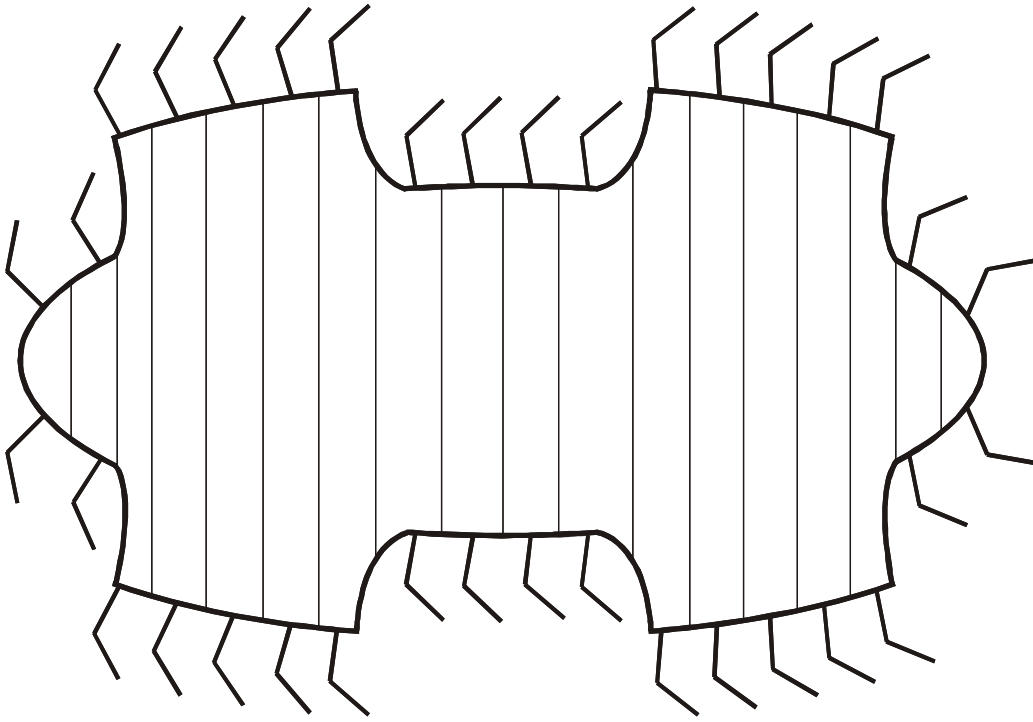
Рисунок 9. Промежуточный этап образования конечностей.
