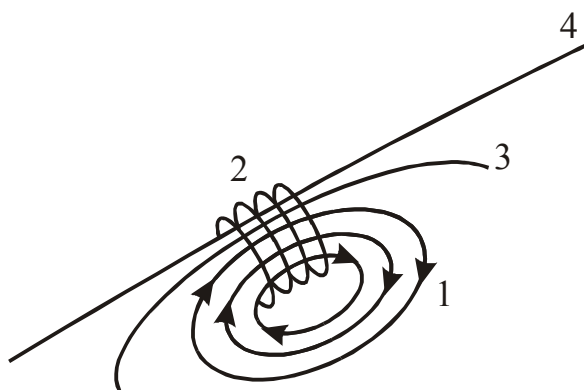
Рисунок 2. Эволюция системы информация-знание-сознание.
