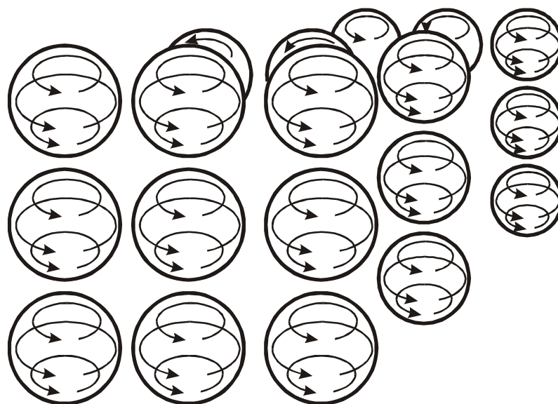
Рисунок 51. N-мерная матрица пространств.
