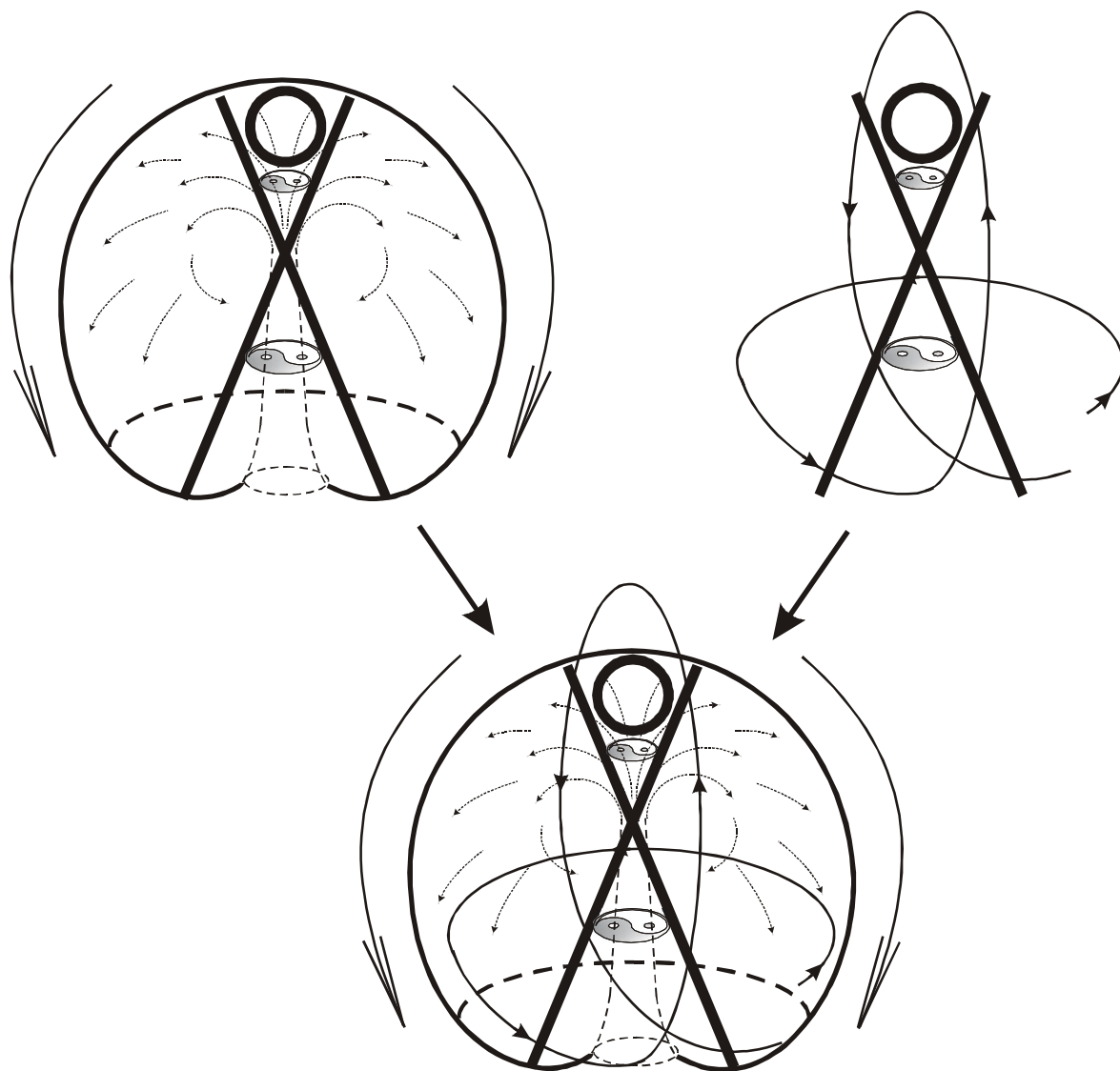
Рисунок 27. В конструкции человека повторяются все основные вселенские принципы построения сложных систем.
