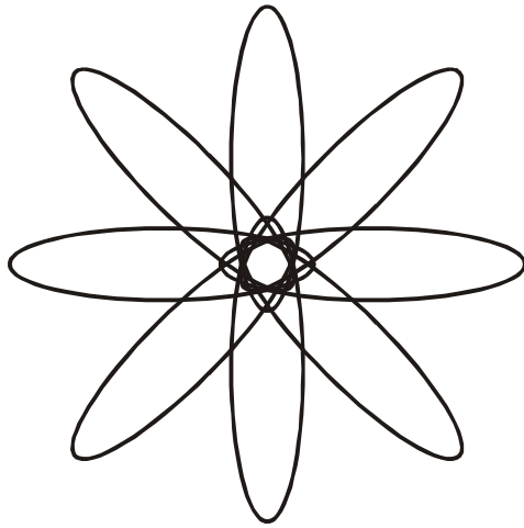
Рисунок 44. Взаиморасположение и траектории пучка параллельных Вселенных вокруг общего центра.
