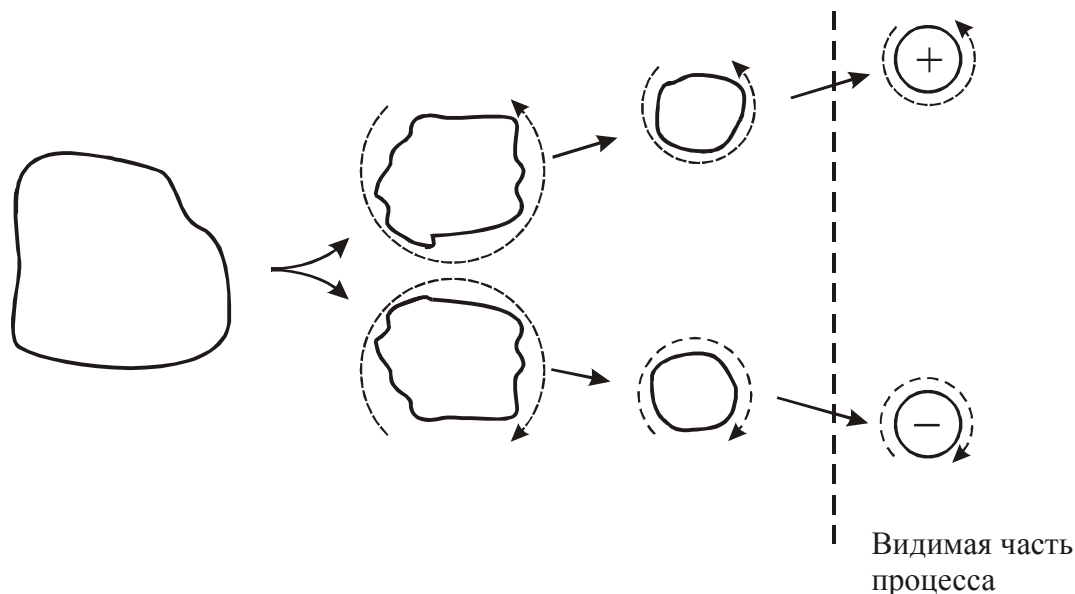
Рисунок 40. Рождение пары частица-античастица. Абсолют создает пары.
