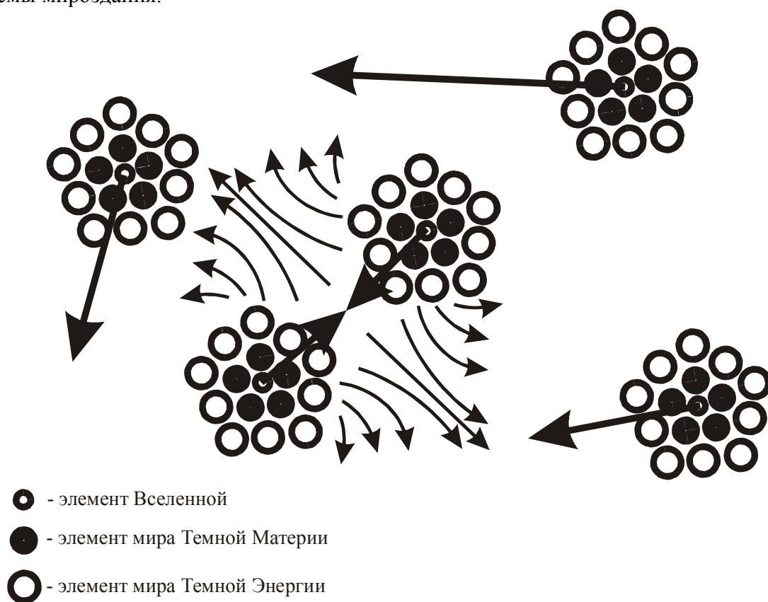
Рисунок 30. Взаиморасположение элементов 3-х миров.
