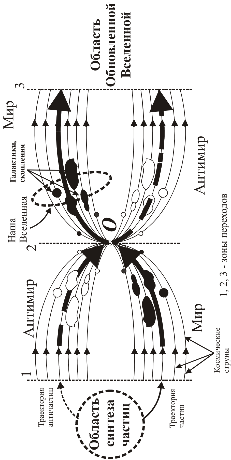
Рисунок 42. Структура параллельных Вселенных.
