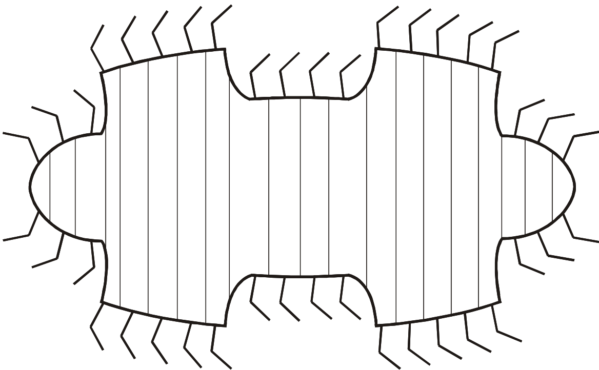
Рисунок 10. Структурирование новых органов.
