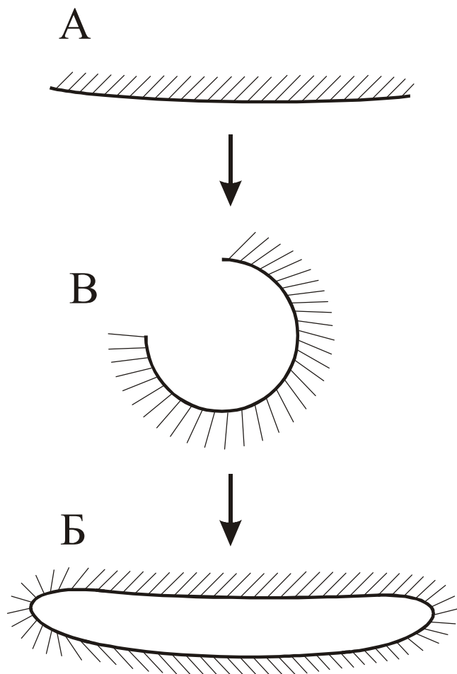
Рисунок 63. Преобразование линейного волнового фронта А в циклический - Б, через промежуточную форму В.
