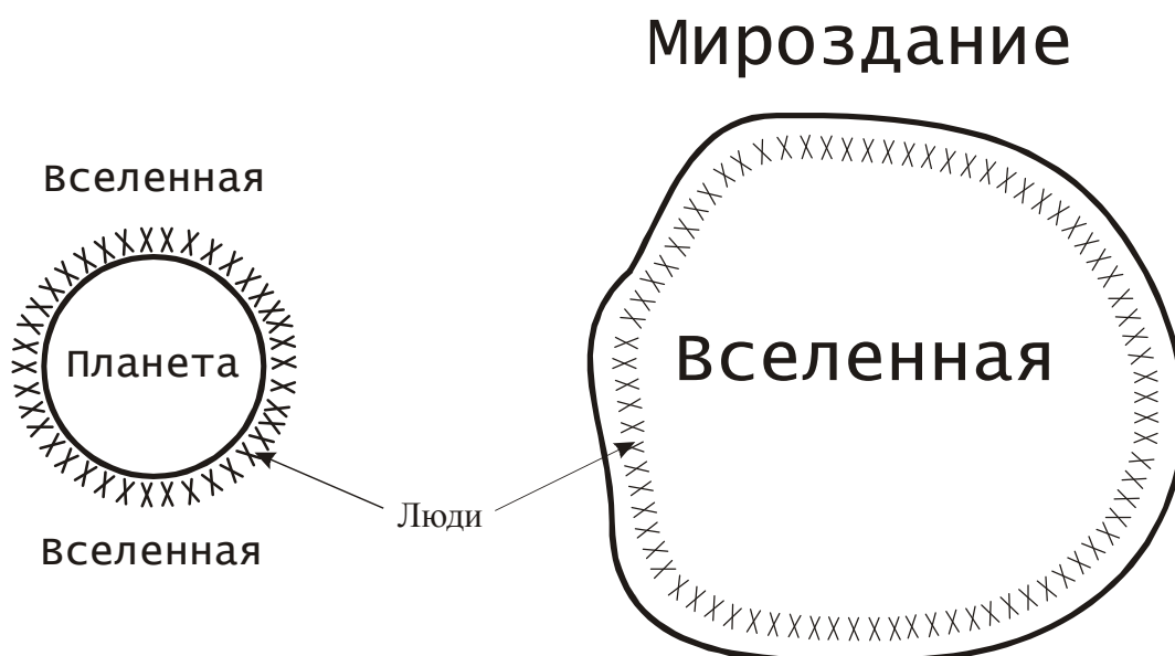
Рисунок 47. Человек - проводник воли Неба во Вселенной, на всех её планетах
